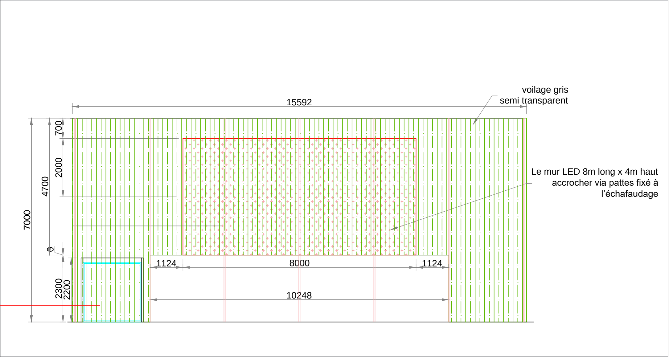
ELEVATION A
